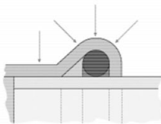
rys. Kierunki nacisku w połączeniu „press”
